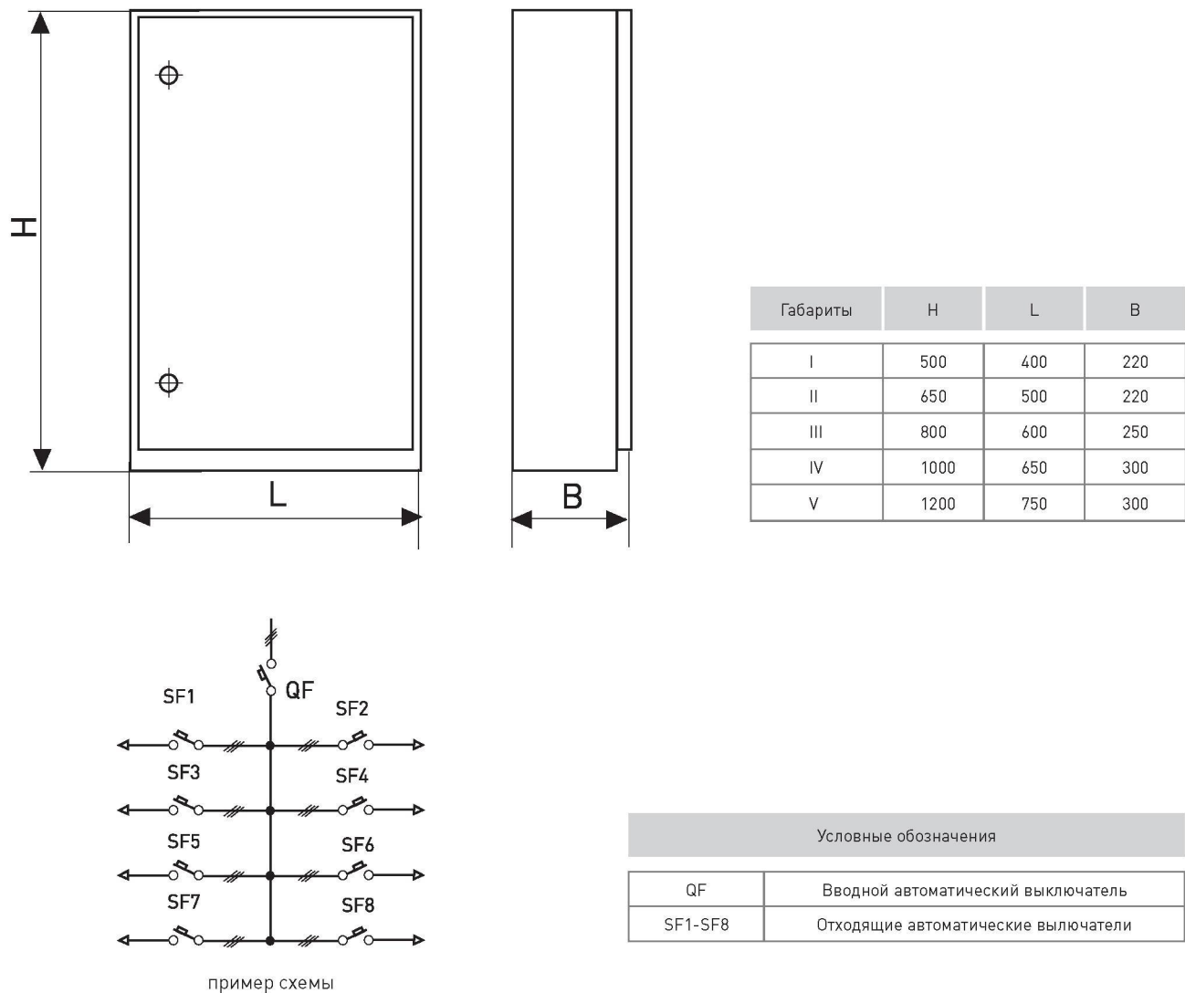
Рис. 6 Общий вид, габаритные размеры и пример схемы шкафа распределительного ПР11
